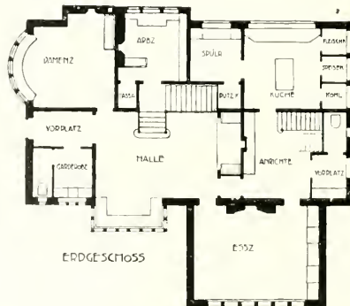
GRUNDRISS ZU OBIGEM LANDHAUS-ENTWURF
