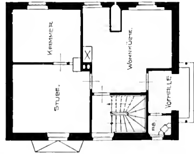
GRUNDRISS DES ERD- UND OBERGESCHOSSES.
