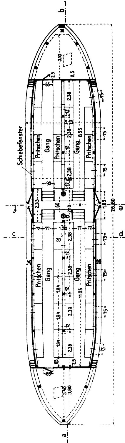
Grundriß
