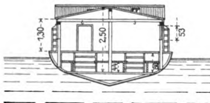
Querschnitt e-d.
