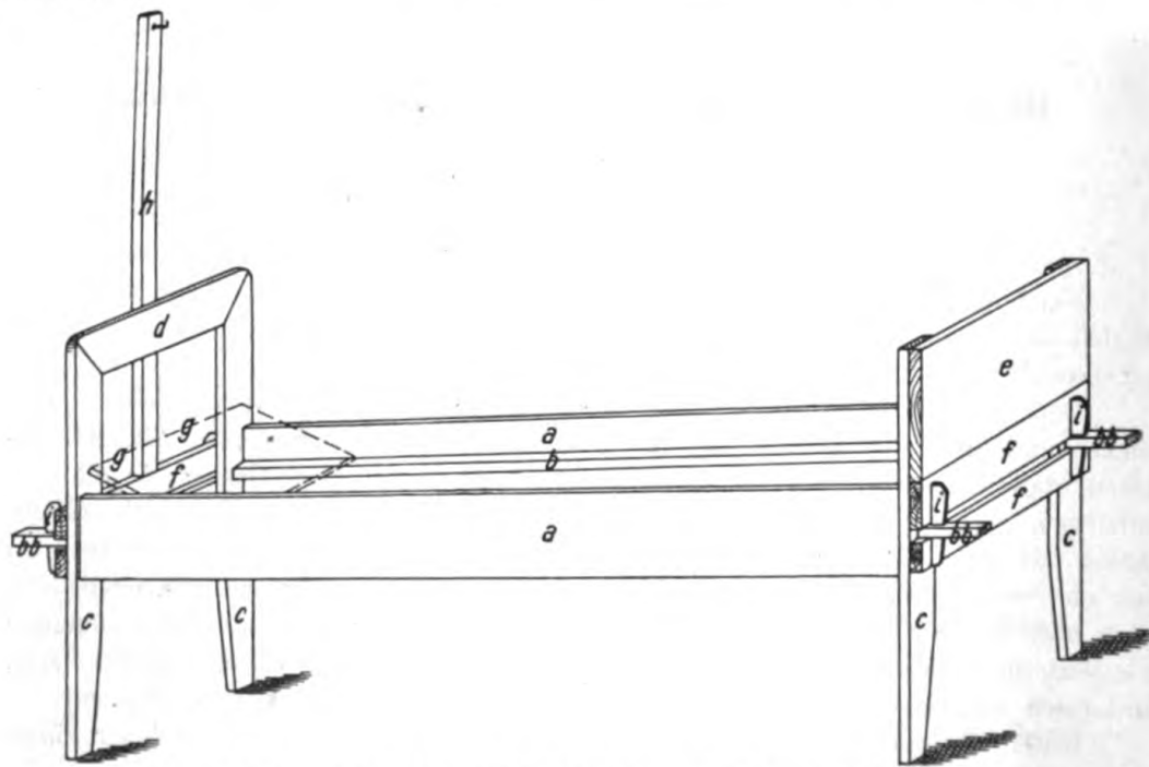
Bild 2. Zerlegbare Feldbettstelle von Holz (verbesserte).
