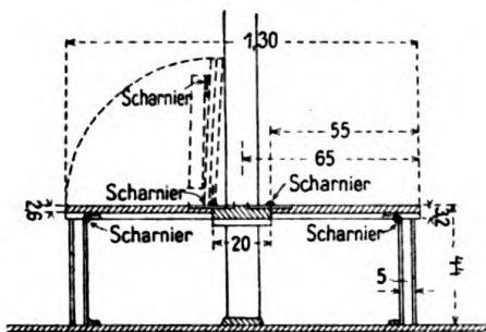
Hochklappen der Pritschen. Detail M. 1 : 36.
