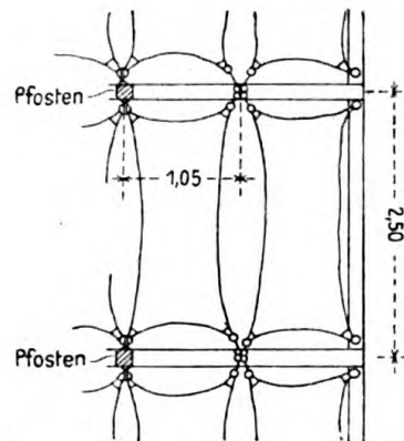
Querschnitt e-f.
