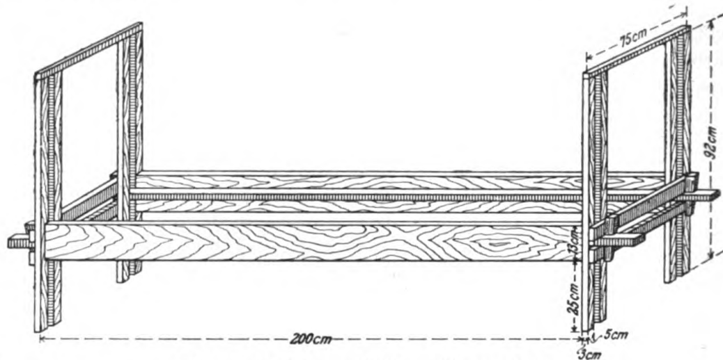
Bild 1. Zerlegbare Feldbettstelle von Holz.
