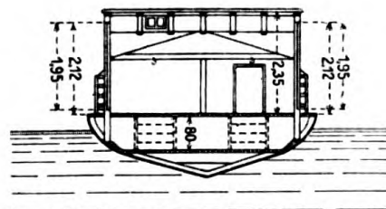
Querschnitt e-f.
