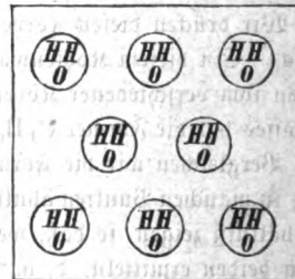
Wasserstoff H_2O .
