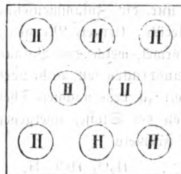
Wasserstoff H
