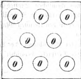
Sauerstoff O
