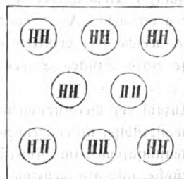
Wasserstoff H_2
