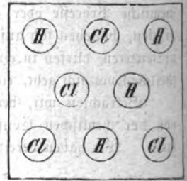
Salzsäure HCl
