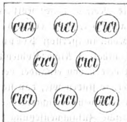
Chlor Cl_2
