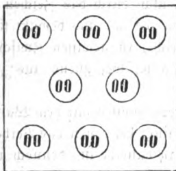
Sauerstoff O_2
