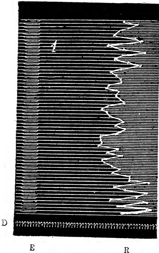
FIG. 74. — Réponse à un signal, d'après PATRIZZI.
