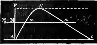
FIG. 23. — Réaction à la force F (schéma).
