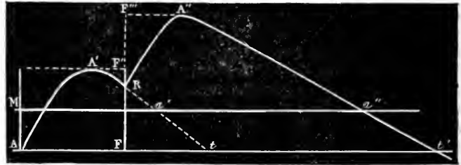
FIG. 21. — Réaction à deux forces successives (schéma).
