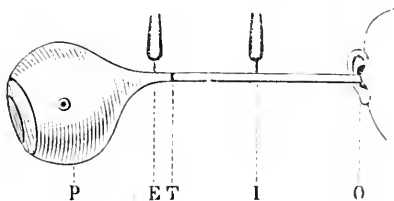
FIG. 78. — Dispositif pour montrer l'effet des tensions du tympan sur l'audition.
