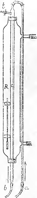
FIG. 27. — Aérotonomètre de FREDERICQ.
