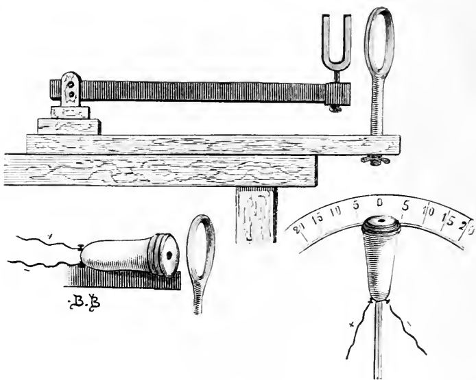
FIG. 75. — Appareil pour mesurer la durée de l'excitation nécessaire à l'audition.
