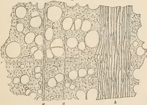
Querschnitt durch Rothbuchenholz. Vergrößerung: 100/1 .
