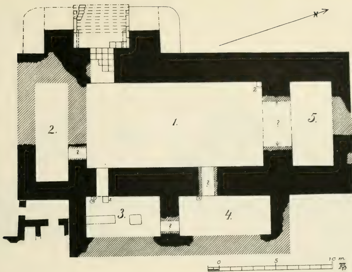
a) SCHEMATISCHER GRUNDRISS DES E-TEMPELS 1:200
