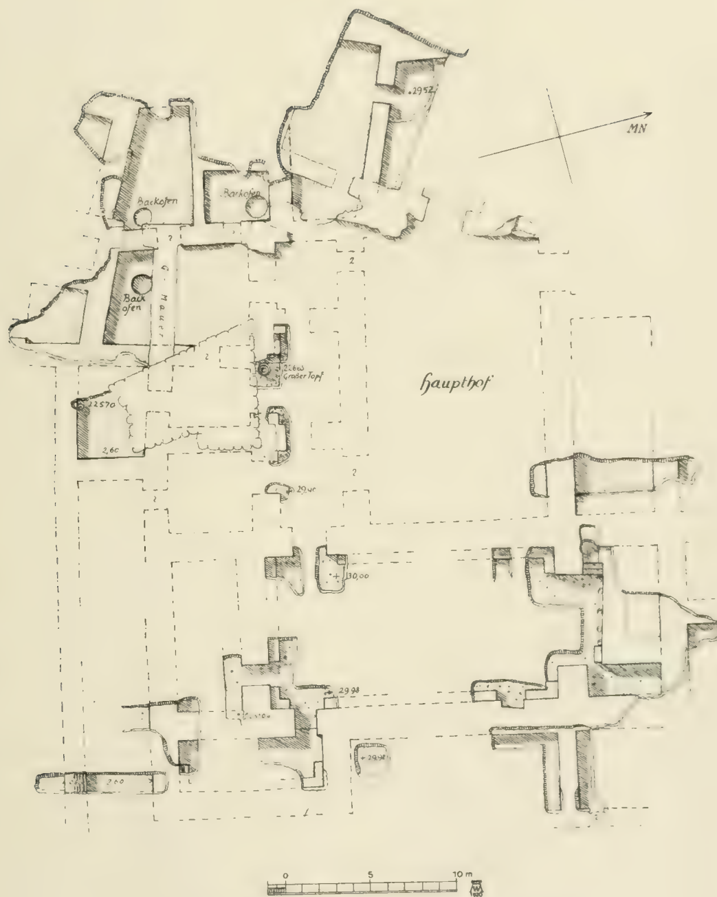
DER H-TEMPEL NACH DER AUSGRABUNG 1 : 200
