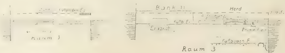
Abb. 73. Querschnitte Ost-West und Süd-Nord durch Raum 3 des E-Tempels.
