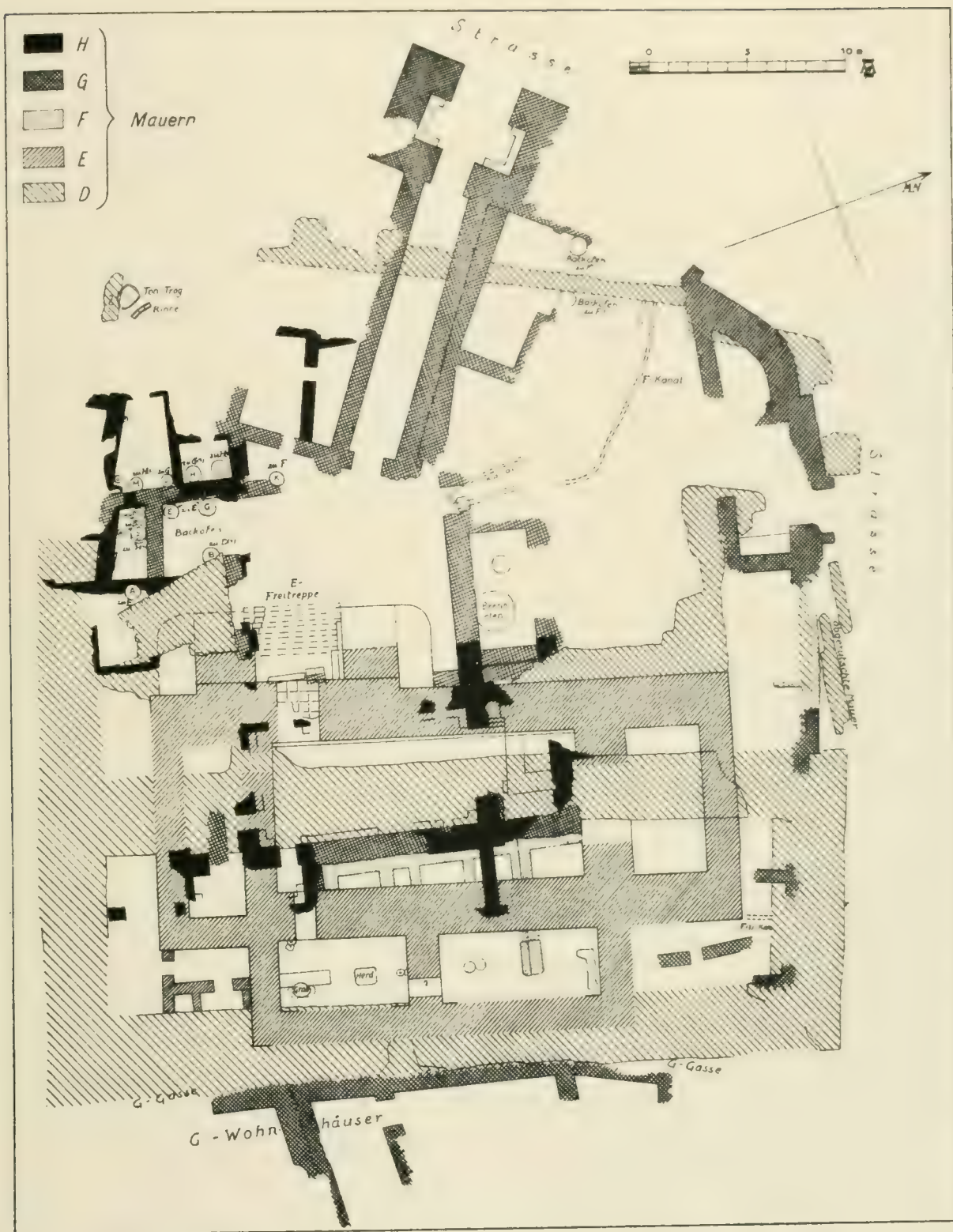
SCHEMATISCHER GRUNDRISS DER ARCHAISCHEN ANLAGEN 1:300
