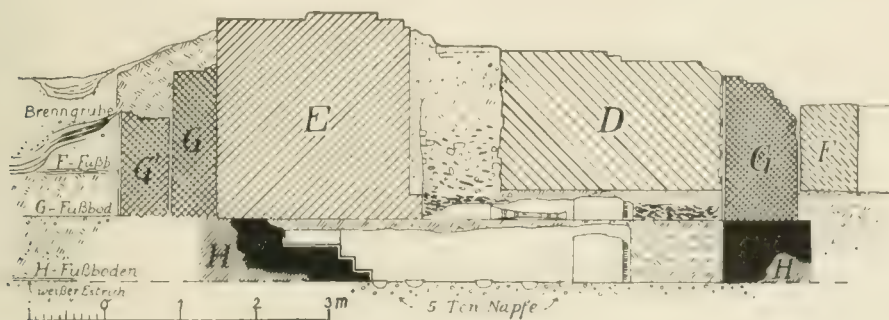
Abb. 10. West-Ost-Schnitt durch das Allerheiligste von H und G. 1:100.
