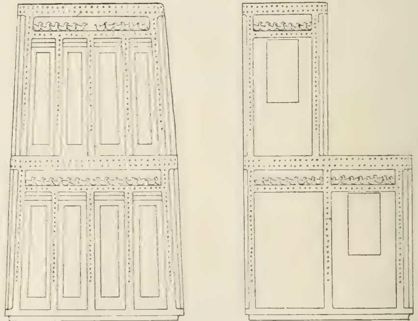
Abb. 8. Tonhäuschen 11 ergänzt. Vorder- und linke Seitenansicht. \frac{1}{8} d. nat. Gr.
