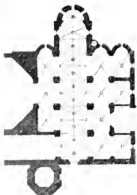
GRUNDRIß DER KIRCHE ST. FELIÚ IN GERONA (Nach Ferencz)
