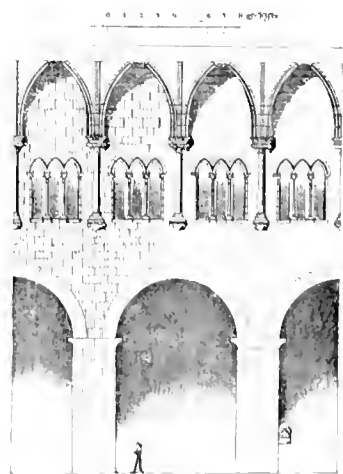
LÄNGENSCHNITT DER KIRCHE ST. FELIÚ IN GERONA (Nach Ferencz)
