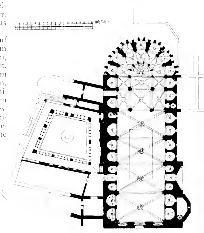
GRUNDRISS DER KATHEDRALE UND DES KREUZGANGES VON GERONA (Nach Ferencz)
