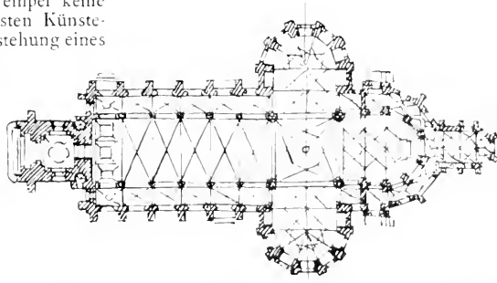
GRUNDRISS DER ST. BERNARDUSKIRCHE IN KARLSRUH
