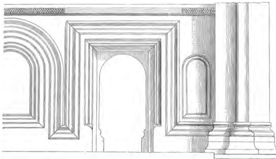
Ansicht des Lettners vom Chor aus. \frac{1}{10} nat. GröÙe.
