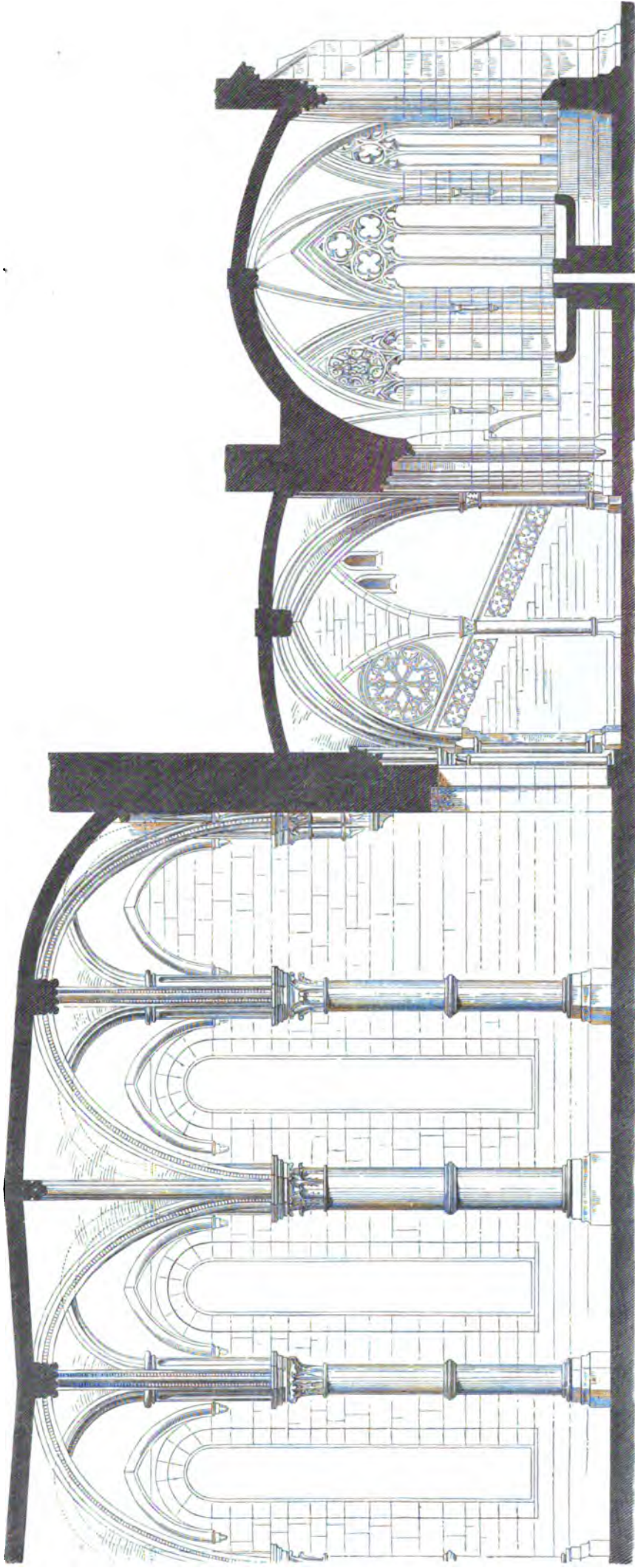
Schnitt durch Porenceforium, Kreuzgang und Brunnenkapelle. 1/100 nat. GröÙe.
