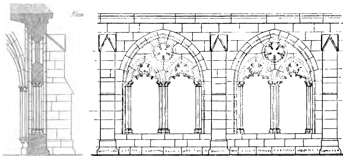
Fenster im Westflügel des Kreuzgangs.
