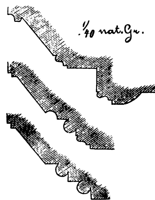
Profile des nördlichen Chorsankers.
