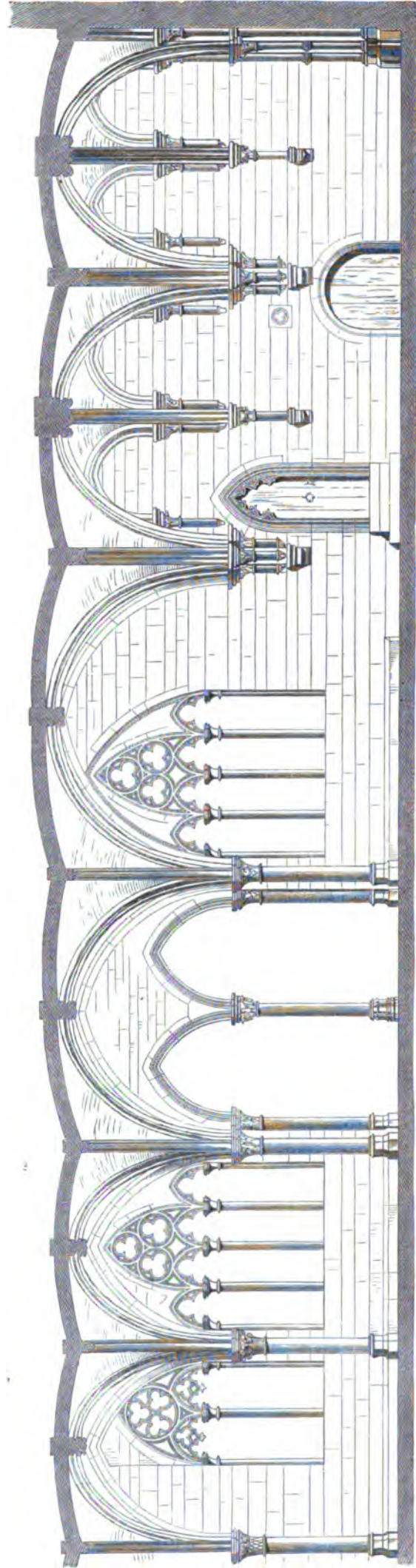
Längenschnitt durch den Pfeiler des Kreuzgangs mit Blick gegen den Kapitelsaal. 1/100 nat. GröÙe.
