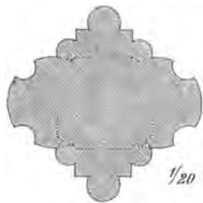
Durchschnitt über dem Kapital einer schwächeren Säule.
