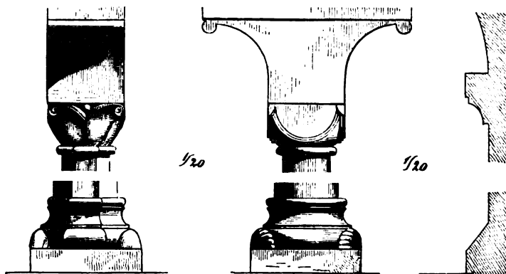
1/20 1/20 1/20 Details vom Arkadengang des Herrenhauses.
