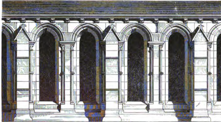
Südllicher Kreuzgangsfügel. 1/100.
