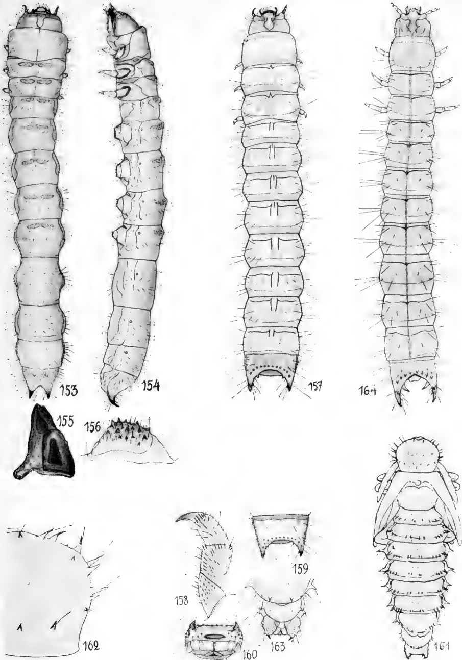
153—156. Calopus serraticornis L. — 157—163. Pytho depressus L. — 164. P. kolwensis C. SAHLB.
