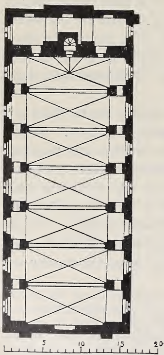
Bild 20. Siegen. Mariä Himmelfahrtskirche. Grundriß.
