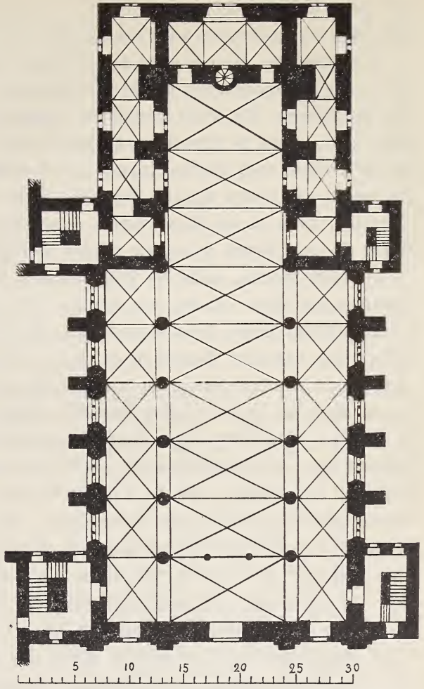
Bild 16. Paderborn. Kirche des hl. Franz Xaver. Grundriß.
