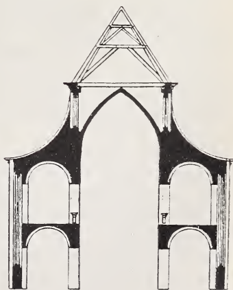
Bild 11. Köln. Idea Moguntina. Querschnitt.
