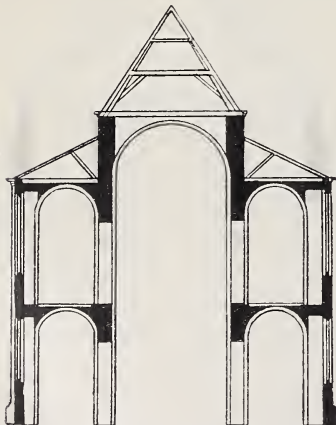
Bild 7. Köln. Idea II Bavarica. Querschnitt.
