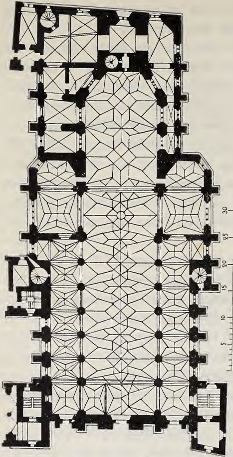
Bild 12. Mariä Himmelfahrtkirche. Grundriß.
