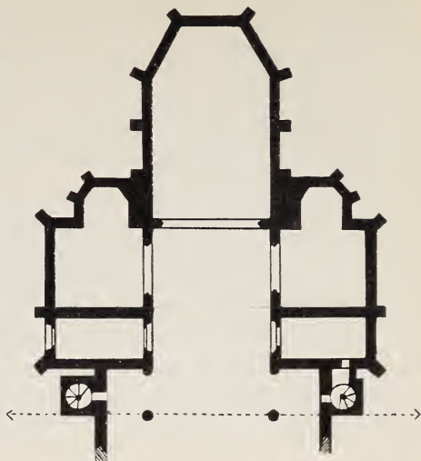
Bild 3. Molsheim. Heutiger Chor. Grundriß.
