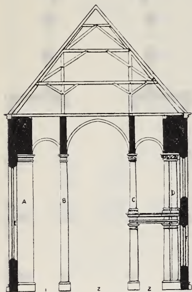
Bild 9. Köln. Idea III Bavarica. Querschnitt.
