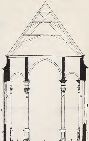
Bild 5. Köln. Idea I Bavarica. Querschnitt.
