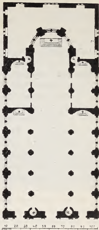
Bild 10. Köln. Idea Moguntina. Grundriß.
