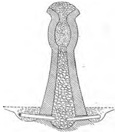
Fig. 4. Durchschnitt desselben.
