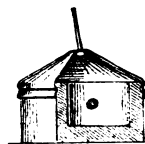
Fig. 20. Aufgeblasener Balg in Orissa. Nach BLANFORD.
