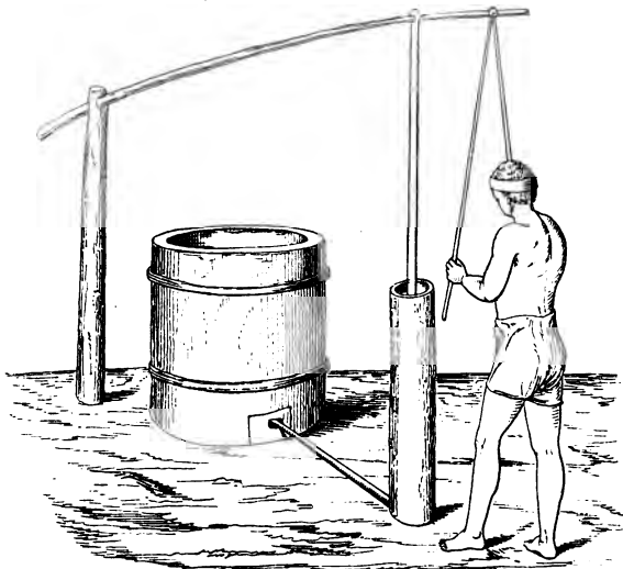
Fig. 24. Eisenschmelze der Dajaks. Nach TEMMINCK.
