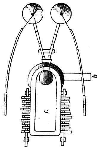
Fig. 19. Eisenofen in Orissa. Obere Ansicht.
