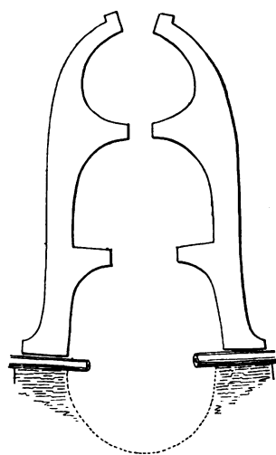
Fig. 6. Berr, Schmelzofen der Bongo. Nach SCHWEINFURTH.
