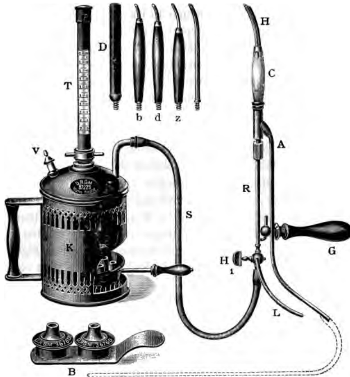
Fig. 14. Instrumentarium zur Atmokaussis nach Pincus.
