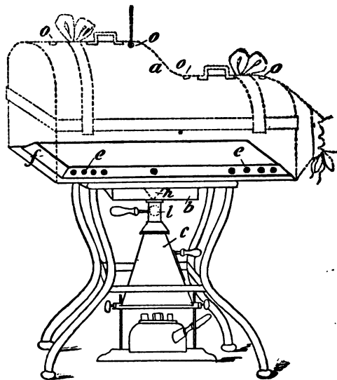
Fig. 8. Derselbe Apparat, Seitenansicht.
