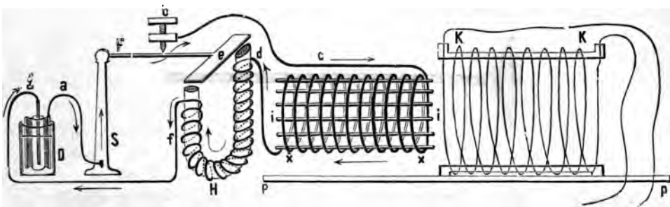
Fig. 60. Schematische Darstellung des Induktionsapparates. Nach Erben.
