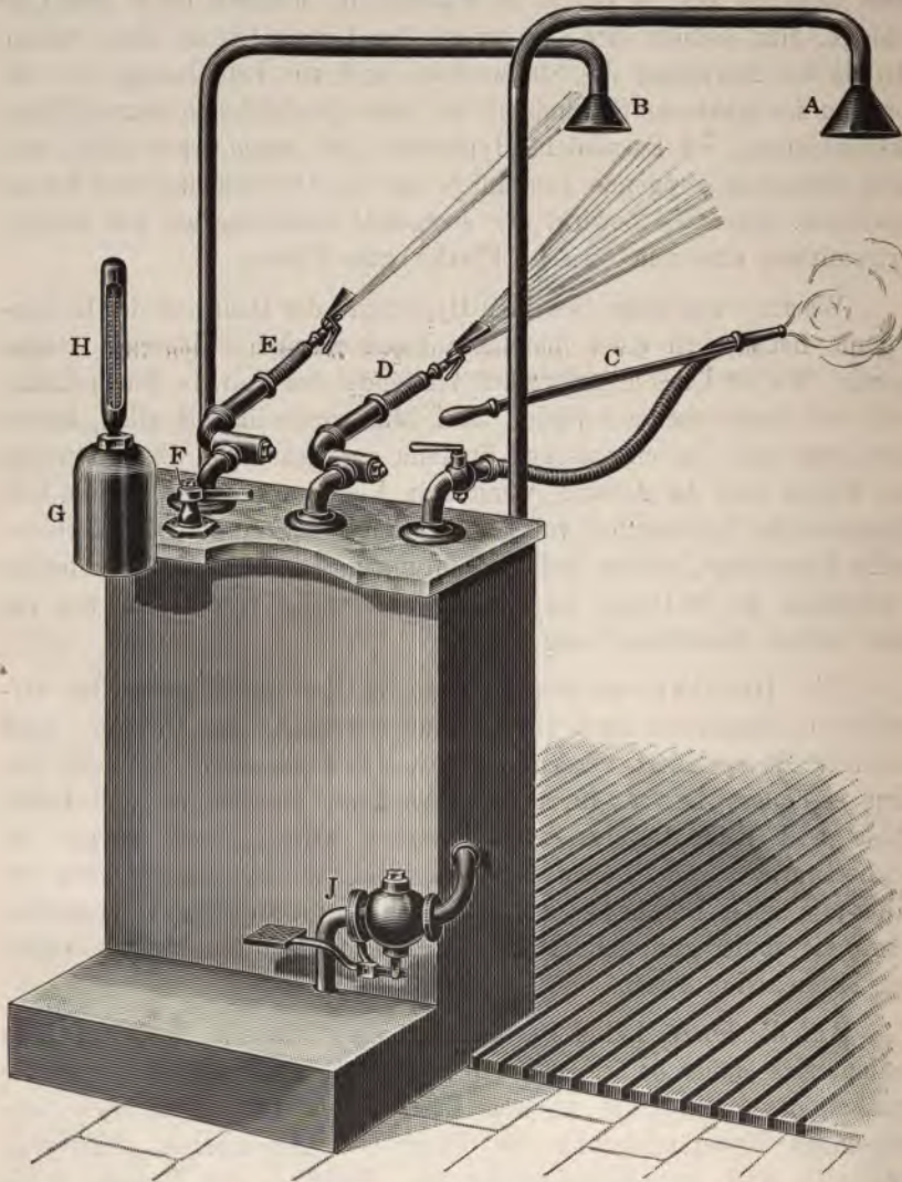
Fig. 12. Dushekatheder nach Winternitz. A. Brause für kaltes Regenbad, regulierbar mit dem Fuße durch das Ventil J. — B. Brause für temperiertes Regenbad, regulierbar durch den Wechselhahn F. — C. strömender Wasserdampf für die schottische Dusche. D. kalte, horizontale Strahl- und Fächerdusche. E. temperierbare horizontale Strahl- und Fächerdusche. G. Mischkessel. H. Thermometer.
