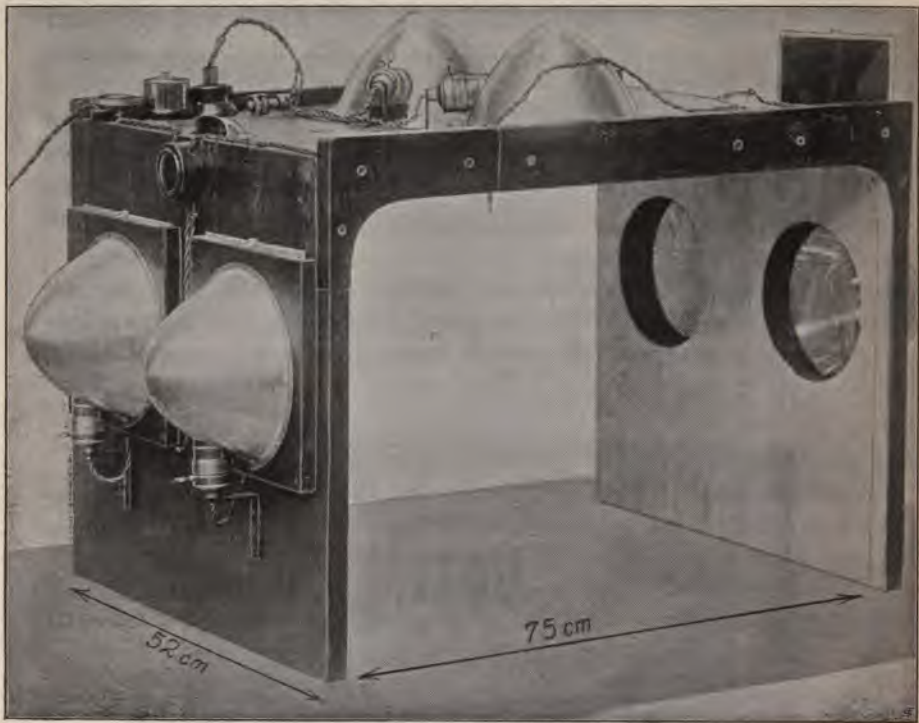
Fig. 4. Elektrisch geheizter Holzsturz.
