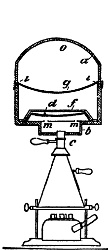
Fig. 7. Schematischer Schnitt durch den Odelgaschen Apparat.
