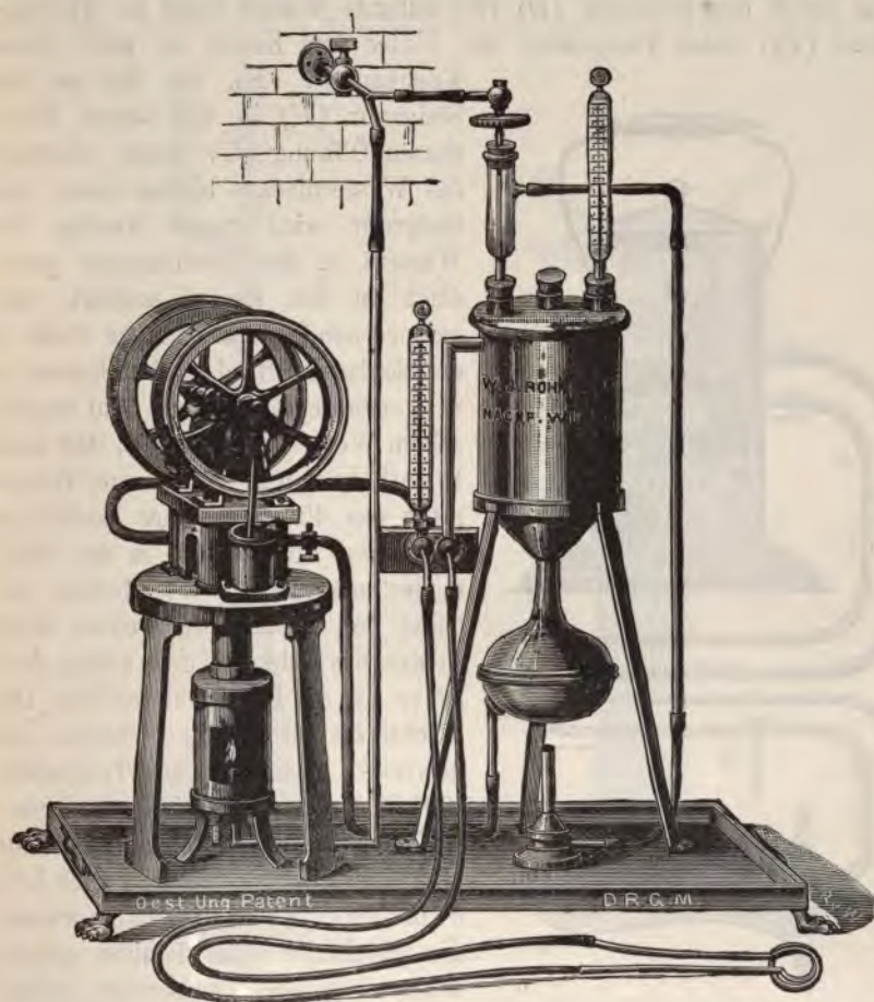
Fig. 20. Hydrothermoregulator nach Ullmann.
