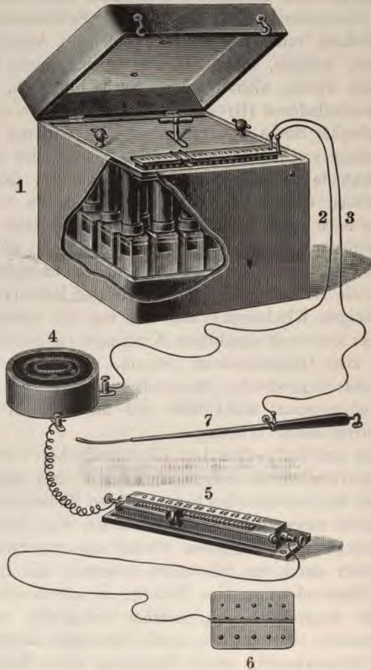
Fig. 55. Apostolis Instrumentarium zur Galvanolyse. Nach Fritsch.
