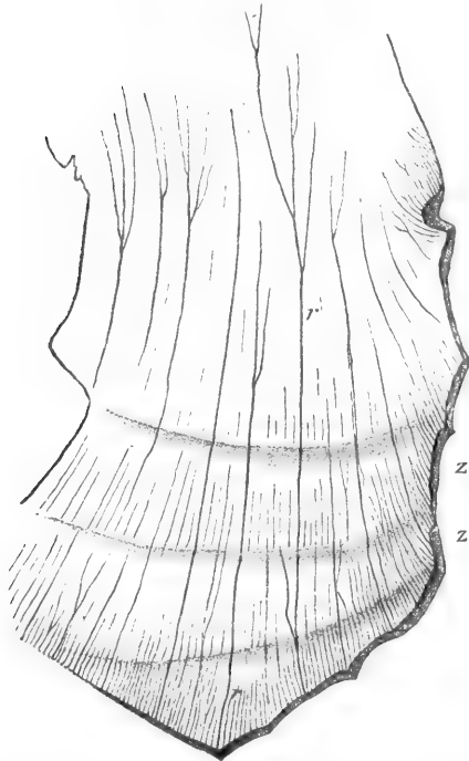
Fig. 9. Vergrößerung 40 mal. Bruchfläche von einem Stück arabischen Gummi. Die Risslinien rr stehen genau oder nahezu senkrecht auf den Zonen ( z ) der Muschelbruchfläche. Nach links ist die Fläche unbegrenzt.
