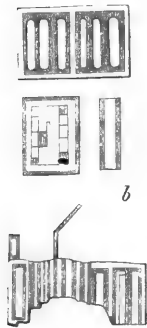
Fig. 89. a Vergr. 300. Wachsschüppchen von der oberen Blattseite von Copernicia cerifera Mart. s s Partien, welche die Spaltöffnungen deckten. b Beobachtet mit Hartnack's Syst. à immers. Nr. 11. Ocul. holost. Stäbchen der Wachsschuppen vom Blatte der Copernicia cerifera . Die schraffirten Partien erscheinen im Mikroskop bläulich, die übrigen röthlich.
