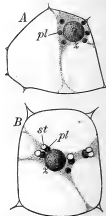
Fig. 94. Vergr. 850. A sehr junge Zelle des Markparenchyms aus dem Rhizom von Canna gigantea . B etwas ältere Zelle. z Zellkern, pl Plastiden (Amyloplasten), welche Stärkekörner ( st ) erzeugen. (Nach A. F. W. Schimper.)
