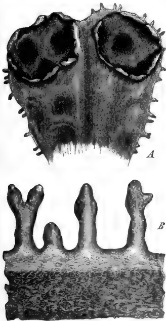
Fig. 137. Cetr. isl. A ein Lappen des Thallus mit zwei Apothecien, vergrößert. B ein Stück vom Rande des Thallus mit vier Spermogonien enthaltenden Wimpern, noch stärker vergrößert. (Nach Luerssen.)
