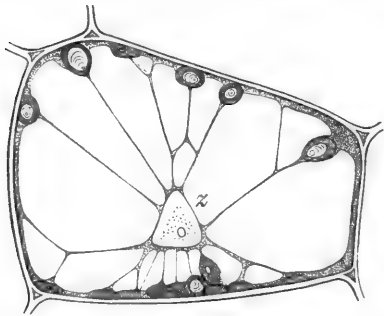
Fig. 92. Vergr. 500. Peripher gelegene Parenchymzelle einer ergrünenden Kartoffelknolle; vom Zellkern z aus strahlen Plasmafäden gegen die (autochthone) Stärkekörner enthaltenden Chlorophyllkörner. (Nach G. Haberlandt.)
