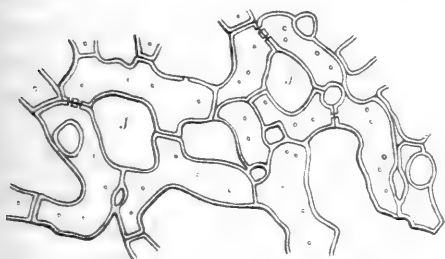
Fig. 141. Vergr. 280. Parenchymzellen der Bassorahgalle. J J Intercellularen.
