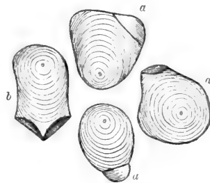
Fig. 106. Vergr. 300. Stärkekörner von Sagus Rumphii . a a Zwillingskörner. b ein Drillingskorn, von welchem die zwei kleinen Körnchen sich abgelöst haben.
