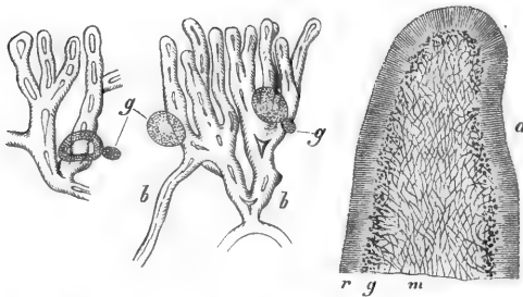
Fig. 128. a Vergr. Contour: 90, Details etwas stärker. Längsschnitt durch die Thallusspitze von Rocella fuciformis . r Rinde. g Gonidien. m Mark. b Vergr. 390. Rindenfasern vom Lager der Rocella fuciformis nach Vorbehandlung mit Ammoniak. g Gonidien. (Nach de Bary).
