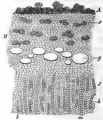
Fig. 152. Vergr. 20. Querschnitt durch die Rinde von Cinchona scrobiculata . A Korksicht. M primäres Rindenparenchym. J Innenrinde. s Sklerenchymelemente (Steinzellen). g Milchsaftschläuche. m Markstrahlen. b b Bastfasern. (Nach A. v. Vogl.)
