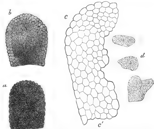
Fig. 90. a b. Vergr. 150. a Drüsen der Fruchthaut von Myrica cordifolia , beim Liegen des Objectes in Wasser, b nach kurzer Einwirkung von Kalilauge. — c. Vergr. 400. Bruchstücke einer Drüse nach längerem Kochen mit Kalilauge. c' Zellen des Hüllgewebes. d bräunliche Zellen der inneren Partie der Drüsen.
