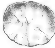
Fig. 139. Vergr. 300. Ligninkörper aus der Nahrungsschicht der Infectoriagalle.
