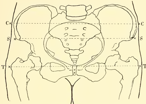
Fig. 49. Weibliches Becken.
