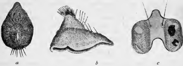
Fig. 10. Eylais infundibulifera .
