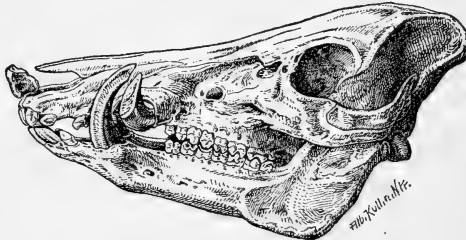
Figur 37. Schädel des Wildschweins. (Aus Schmeil, Leitfaden d. Z.)
