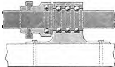
Abb. 409. Kugellager für Schiffsschrauben, 1862.
