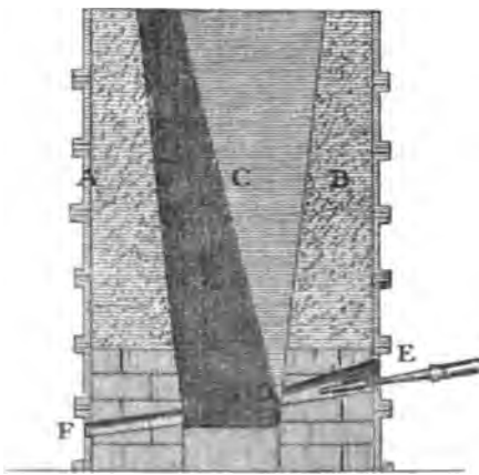
Abb. 159. Wilkinsofen 1794. Nach Repert. of arts, Bd. 1, S. 370.
