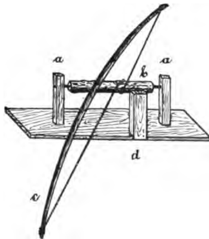
Abb. 145. Der Fiedelbogen zum Antrieb einer einfachen Universalmaschine; rekonstruiert vom Verfasser. Auf dieser Maschine kann man abdrehen, ausdrehen (ausbohren), Löcher bohren, Löcher oder Verzierungen einschleifen, abschleifen, fräsen, drücken, polieren usw. Man braucht nur die betreffenden Werkzeuge in das eine Ende der Achse zu befestigen.
