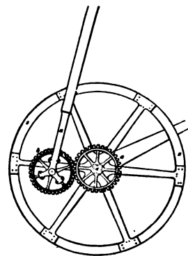
Abb. 403. Planetenrad von 1781, nach der Patentschrift.
