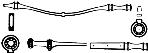
Abb. 405. Kugellager von 1794, nach der Patentschrift.
