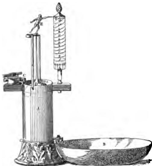
Abb. 778. Wasseruhr des Ktesibios nach der Rekonstruktion von Oskar Hülcker, in: M. C. P. Schmidt, Antike Wasseruhr, 1912, Fig. 24. Jüngst wurde dem Deutschen Museum in München die Rekonstruktion einer Wasseruhr zum Geschenk gemacht. Vgl.: Nachtrag.
