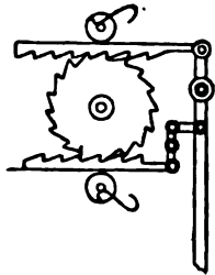
Abb. 588. Schaltwerk von Leonardo, um 1494, nach Beck.
