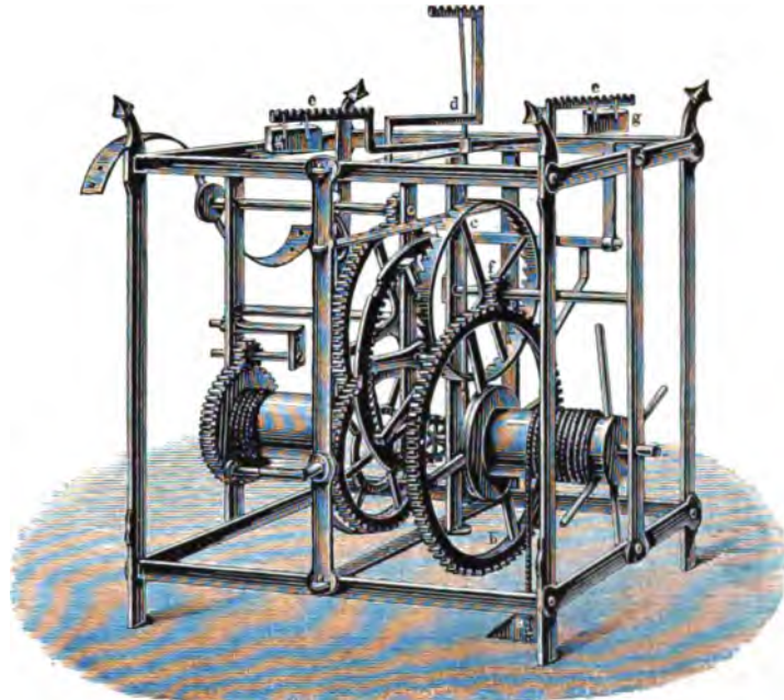
Abb. 776. Londoner Turmuhr, angeblich vom Jahre 1348.
