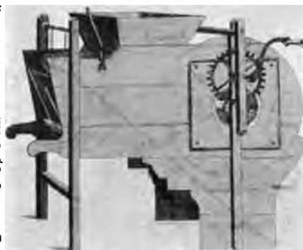
Abb. 692. Siebmaschine, 1760.
