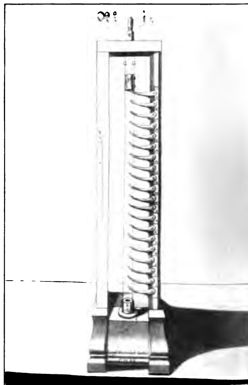
Abb. 601. Schießpulverprober, nach Furttbach 1627.
