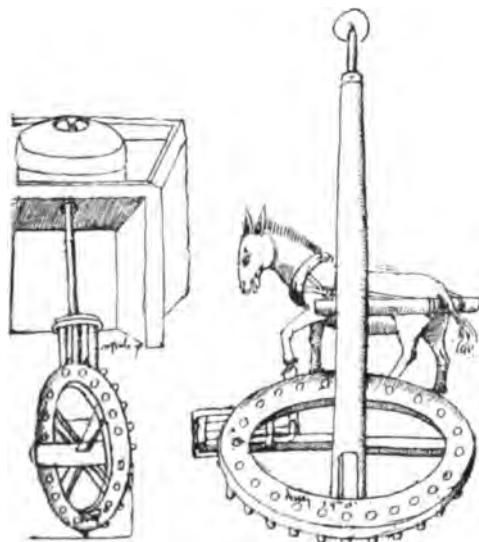
Abb. 320. Göpel (rechts) zum Antrieb einer Mühle (links) unter Anwendung einer unterirdisch geführten Achse, nach Mariano, um 1438.
