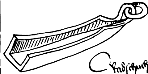
Abb. 356. Hemmschuh, nach U. Besanitzer, 1486, Bl. 15 v.
