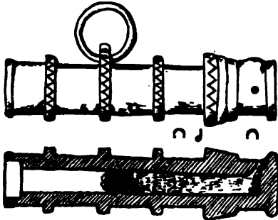
Abb. 282. Ansicht und Schnitt einer ungeschäfteten Klotzbüchse aus Rom. Sammlung Forrer.
