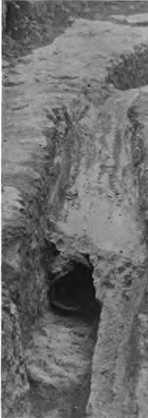
Abb. 577. Kupferne Rinne in Mörtel eingebettet, um 2500 v. Chr., nach Borchardt.
