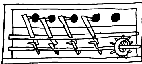
Abb. 717. Stampfe um 1430.
