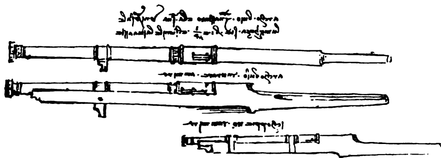
Abb. 284. Hakenbüchsen und ein kurzes, geschäftetes Rohr, nach Leonardo da Vinci um 1500.
