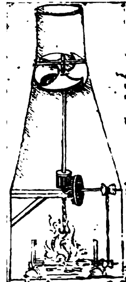
Abb. 98. „Rauchhansel“, Bratenwender mit Warmluftturbine nach Leonardo, um 1500.
