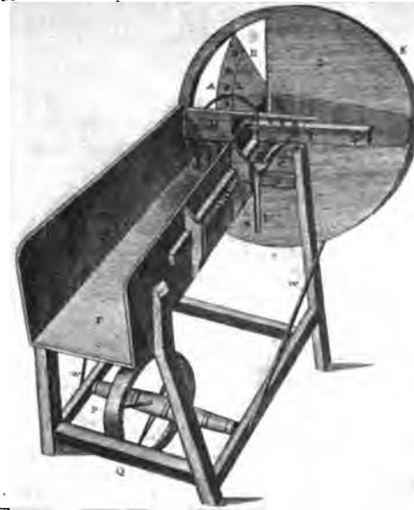
Abb. 329. Englische Häcksellade mit rotierendem Messer, um 1768.
