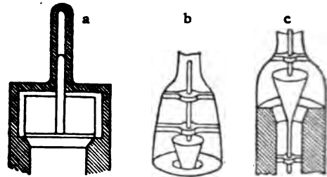
Abb. 332. Ventile nach Leonardo da Vinci.
