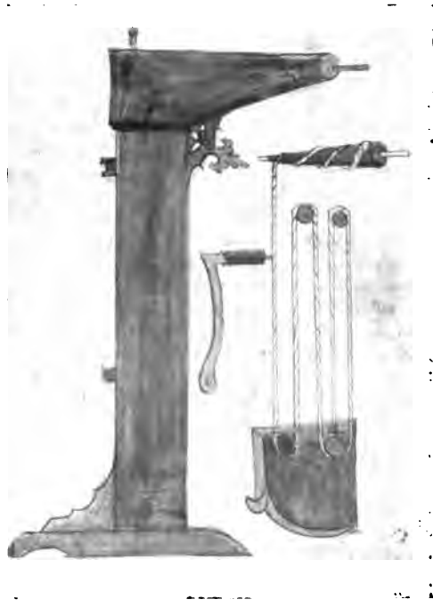
Abb. 21. Armbrustwinde mit konischer Seiltrommel, nach Kyeser, 1405.
