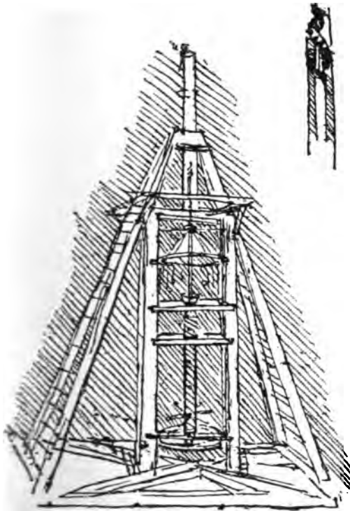
Abb. 97. Große Bohrmaschine für Holzrohre, nach Leonardo um 1500.
