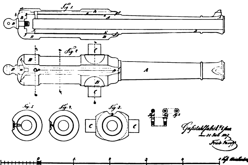
Abb. 263. Die Zeichnung zum preußischen Patent, von Alfred Krupp gezeichnet. Nach dem Originalpatent (Vgl.: F. M. Feldhaus, in: Prometheus 1912, S. 1213).
