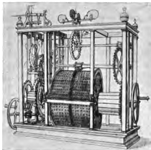
Abb. 318. Zeichnung des Darmstädter Glockenspiels, von 1671.
