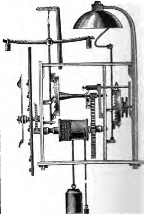
Abb. 775. Türmeruhr, um 1392, im German. Museum Nürnberg. Nach Speckbart.
