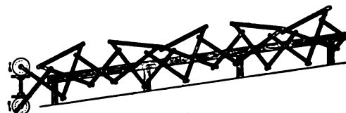
Abb. 535. Schwingrinnen des Turriano in Spanien 1568—1648.
