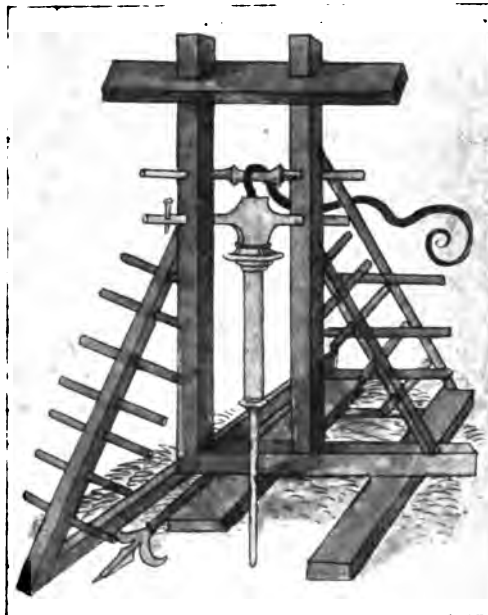
Abb. 93. Fallbohrer um 1540.
