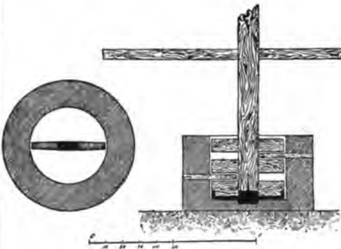
Abb. 392. Rekonstruktion einer römischen Knetmaschine, nach Blümner.
