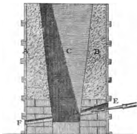
Abb. 159. Wilkinsofen 1794. Nach Repert. of arts, Bd. 1, S. 370.
