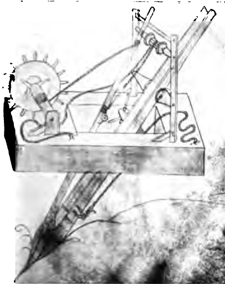
Abb. 48. Stangenbagger, nach Fontana, um 1420.
