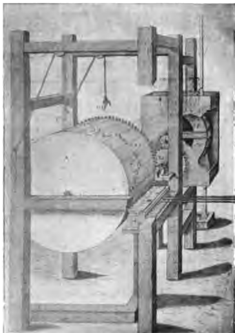
Abb. 505. Orgel mit Stifwalze und Antrieb durch Wasserrad, nach de Caus, 1615.
