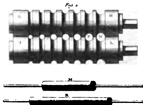
Abb. 798. Röhrenwalzwerk, von Fayolle, 1728. Nach Machines approuvées .
