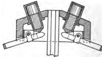
Abb. 267. Schnitt durch die Luftzylinder des Geschützes von Philon; nach: Beiträge zur Gesch. d. Technik , 1912.
