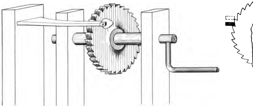
Abb. 872. Rekonstruktion einer einzähniigen Säge zum Tauschieren nach der Beschreibung von Theophilus um 1100.
