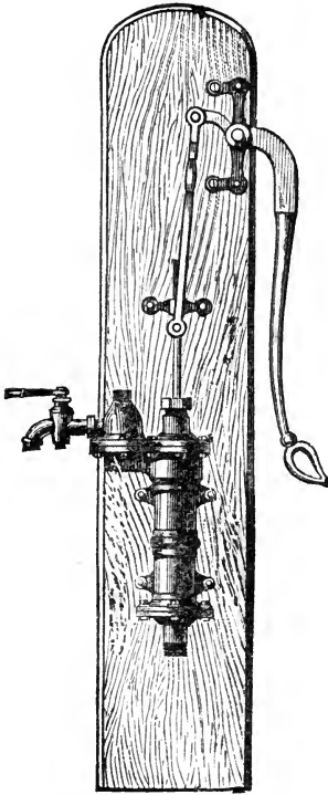
FIG. 347.—Lever pump.
