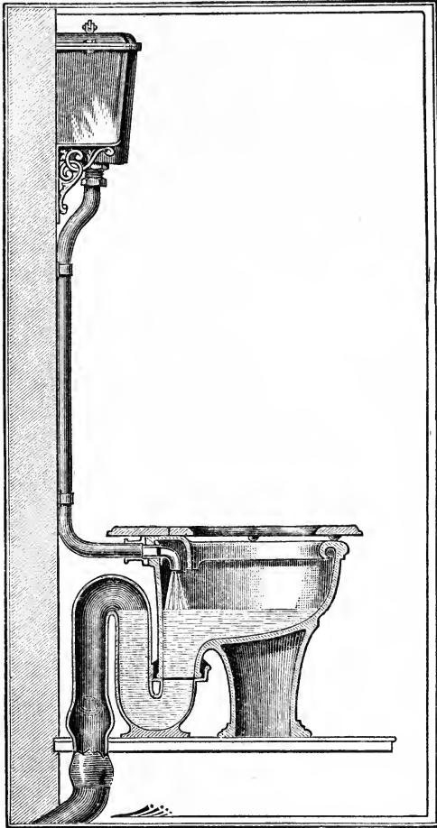
FIG. 180.—Syphonic closet.
