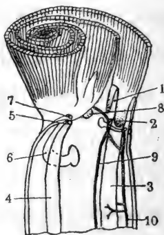
圖 17. 筲蟲 解剖圖
