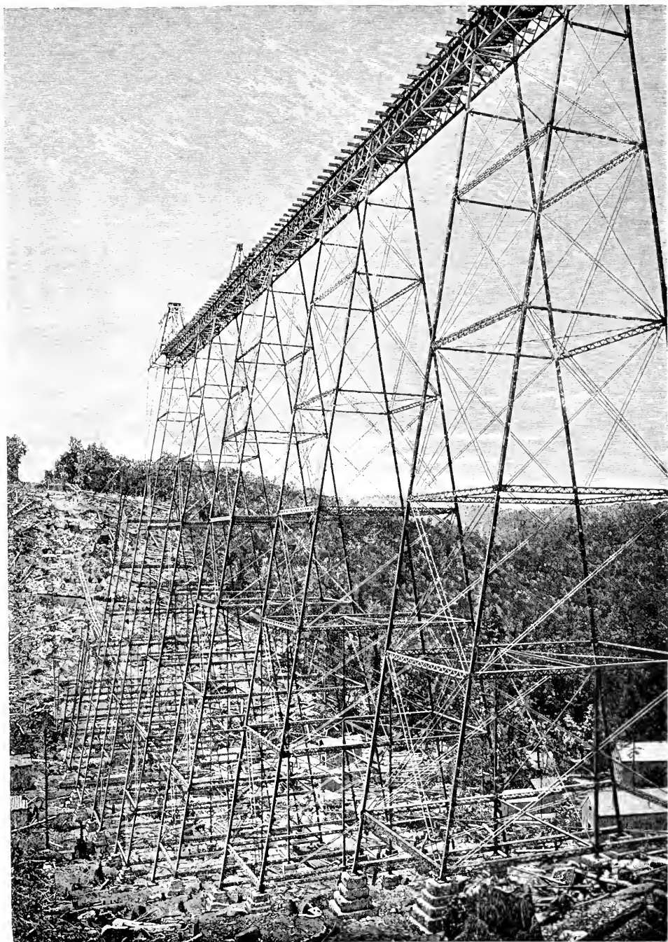
Adolf Bonzanos Kinzua-Brücke während ihres Baus.
