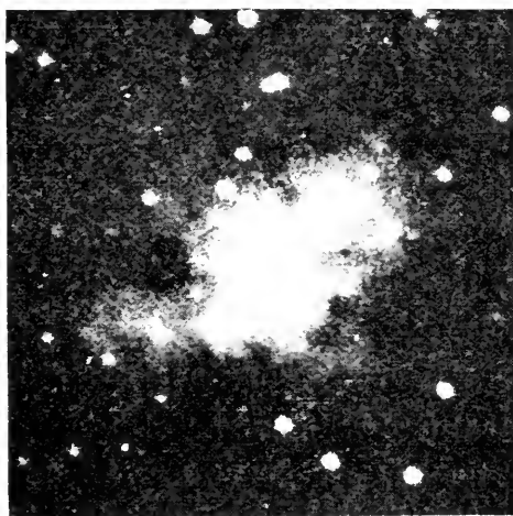
Fig. 3.—THE CRAB NEBULA (n.g.c. 1952; in Taurus).
