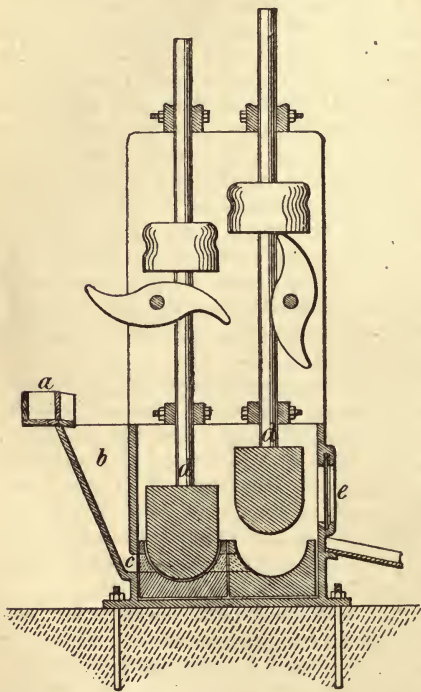
FIG. 173.—TIN STAMP.
