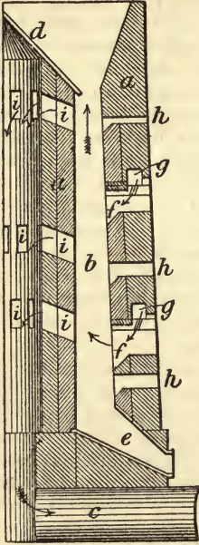
FIG. 146.—DESULPHURISING KILN.
