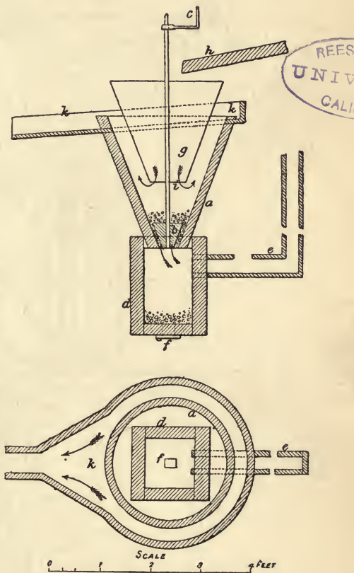
FIG. 73.—FRONGOCH CLASSIFIER.
