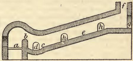
FIG. 148.—MEXICAN SERPENTON.
