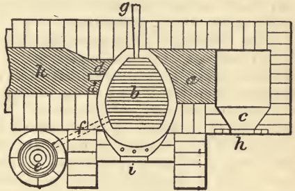
FIG. 156.—ENGLISH CUPEL.
