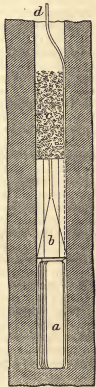
FIG. 8.—TAMPING PLUG.
