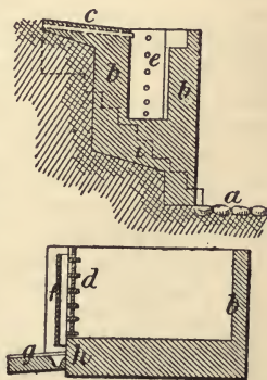
FIG. 171.—LAVADERO.
