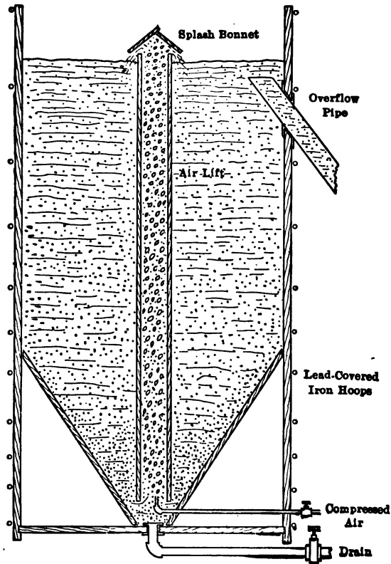
FIG. 4.—Pachuca agitator
