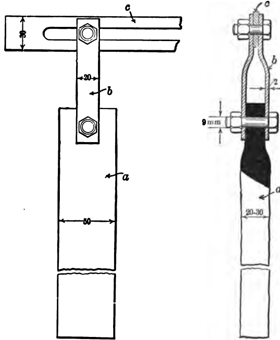
FIG. 22.—Anode connections at Förfurt
