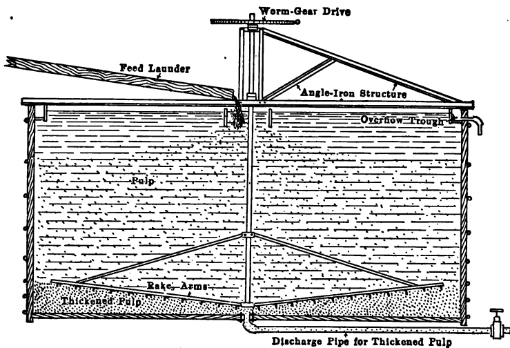
FIG. 5.—Dorr thickener
