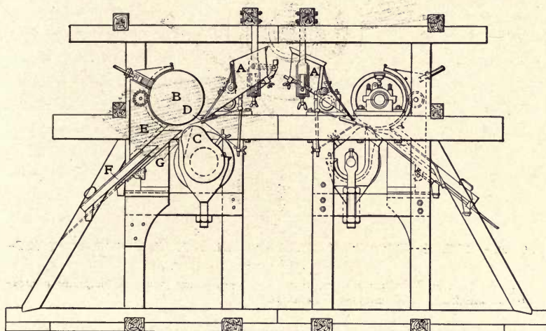
FIG. 37.—MECHERNICH SEPARATOR.
