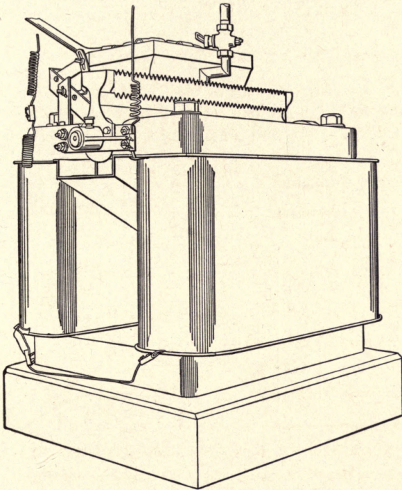
FIG. 23.—THE HUMBOLDT WET SEPARATOR.
