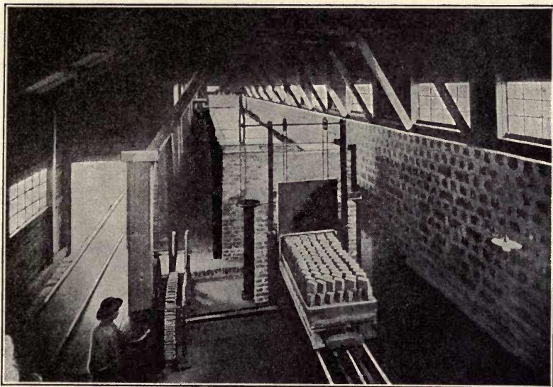
FIG. 58.—BRIQUETTING FURNACE AT GULDSMEDSHYTTAN.
