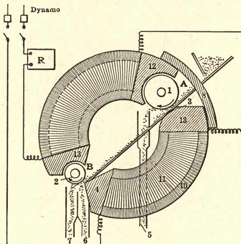
FIG. 44. — THE UBALDI SEPARATOR.
