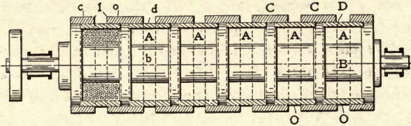
FIG. 1. Longitudinal Section
