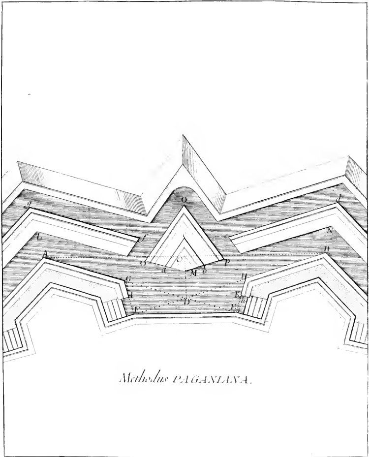
Fig: Archit: Milit: Tab: III.
