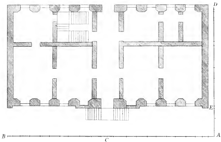
Fig: Archit Civil: Tab: XV.
