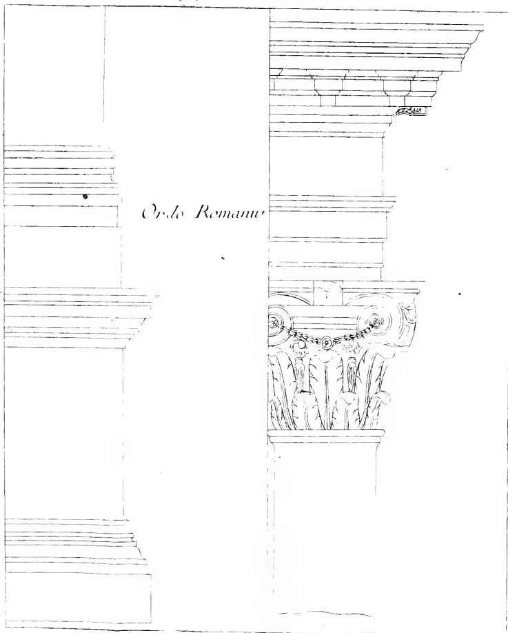
Fig: Archit: Tab: VII
