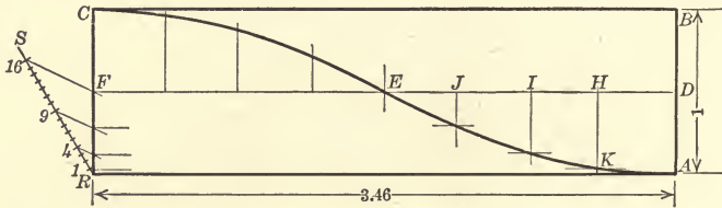
FIG. 25.—PARABOLA
