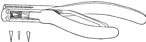
FIG. 485. Point punch
