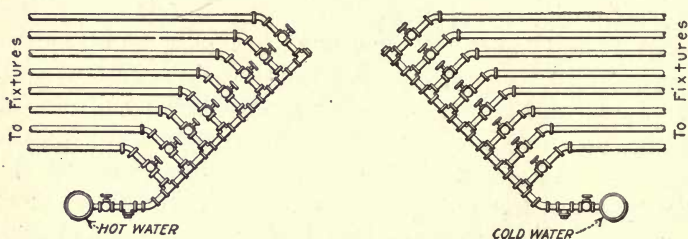
FIG. 70.—“Banjo.”
