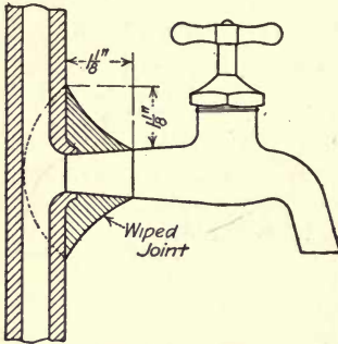
FIG. 32.—Bib.
