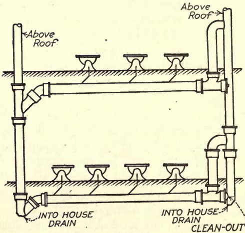
FIG. 55.—Circuit vent.
