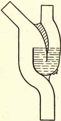
FIG. 62.—Flask trap.
