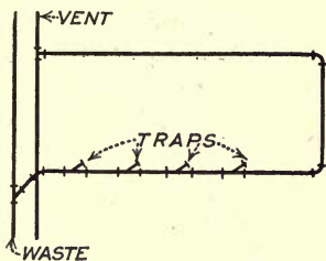
FIG. 56.—Loop vent.
