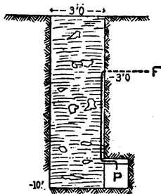
PLATE 9a.—Land mine.
