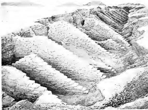
FONDAMENTA O PARETI DI SOSTEGNO DI UN EDIFICIO SOTTOSTANTE A UN CIMITERO.
