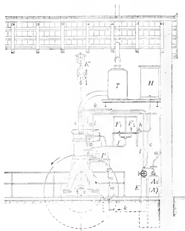
DISPOSIZIONE GENERALE DELL'INSTALLAZIONE DI UN MOTORE DIESEL DA 40 H. P.
