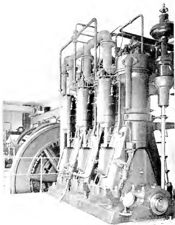
IMPIANTO ELETTRICO CON MOTORE DIESEL FI QUATTRO CILINDRI, TIPO A QUATTRO TEMPI.
