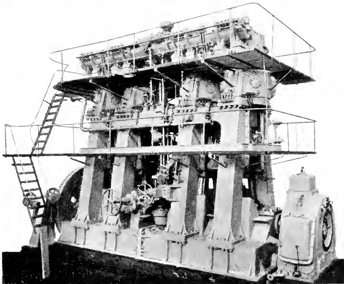
IN ALTO: GRANDE MOTORE DIESEL, TIPO FISSO — IN BASSO: LO STESSO, TIPO MARINO.
