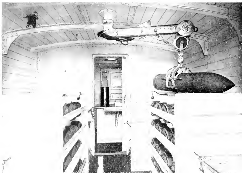
IRENO-BATTERIA PER DIFESA COSTIERA - INTERNO D'UN VAGONE PER MUNIZIONI.
