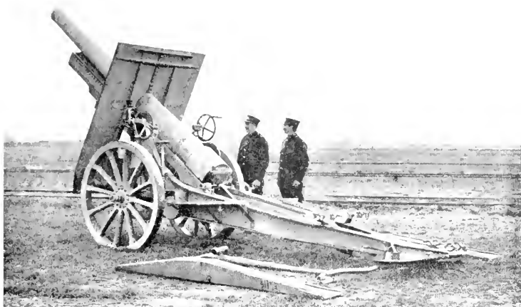
CANNONE SCHNEIDER, DA ASSEDIO, DA 162 MM., A TIRO RAPIDO, PER L'ESERCITO RUSSO.
