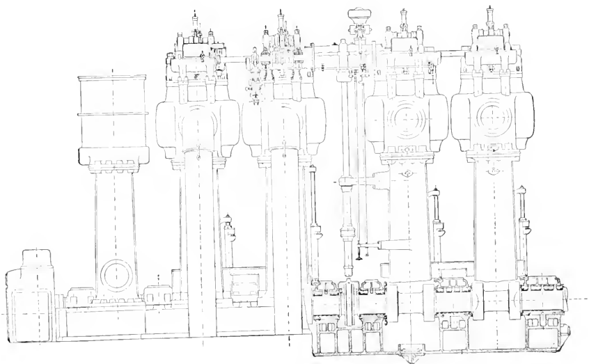
MOTORE DIESEL FISSO, TIPO A DUE TEMPI.
