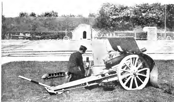
CANNONE SCHNEIDER, DA MONTAGNA, DA 75 MM., A TIRO RAPIDO.
