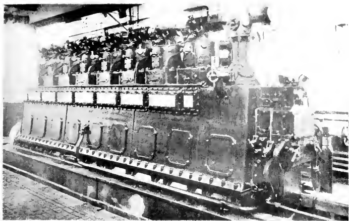
MOTORE DIESEL A DUE TEMPI (TIPO NORIMBERGA) DI 1000 CAVALLI, PER SOTTOMARINI.
