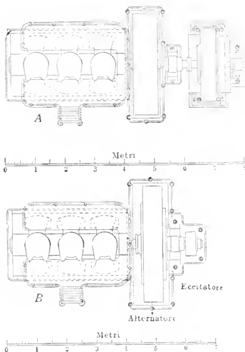
SPAZIO OCCUPATO DA UN MODERNO MOTORE DIESEL DI 300 HP.
