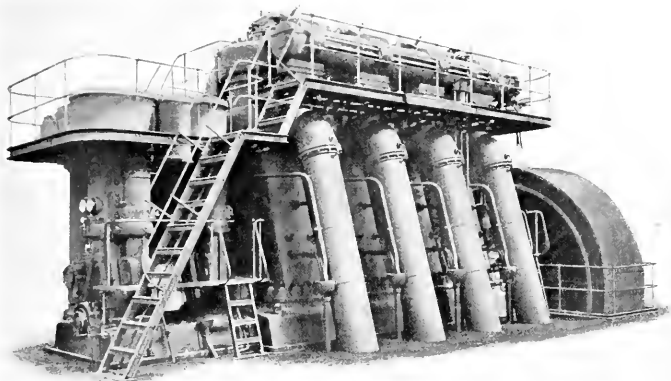
MOTORE DIESEL A DUE TEMPI DI 2000 HP.
