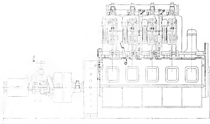
MOTORE AD OLIO PESANTE DI 1000 HP.
