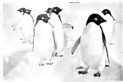
FIG. 8. PINGUINI D'ADELIA.
