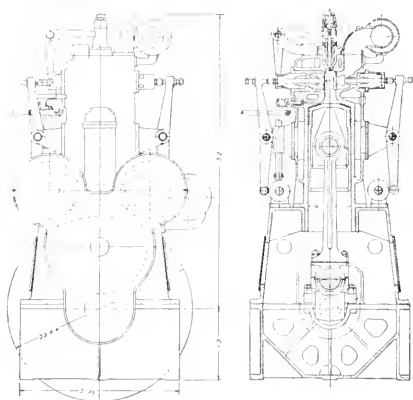
VISTA DI LESTA E SEZIONE DI UN MOTORE DIESEL DA 100 HP.
