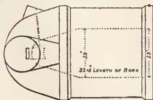
FIG. 22.—13-inch Mortar.
