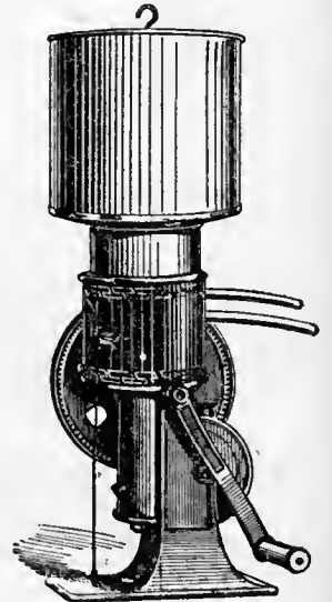
FIG. 18.—Hand-Separator.
