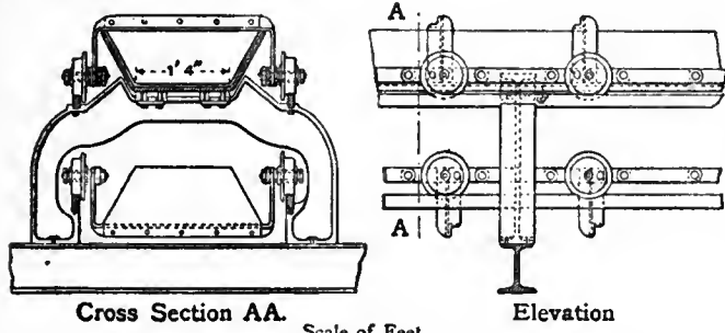
FIG. 12.—Wild Coke Conveyor.
