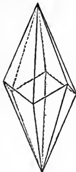
FIG. 68.—Scalenohedron.
