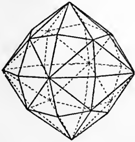
FIG. 24.—Hexakis-octahedron.
