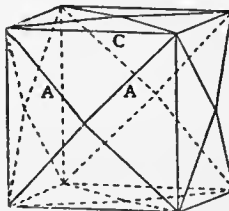
FIG. 21.—Tetrakis-hexahedron.
