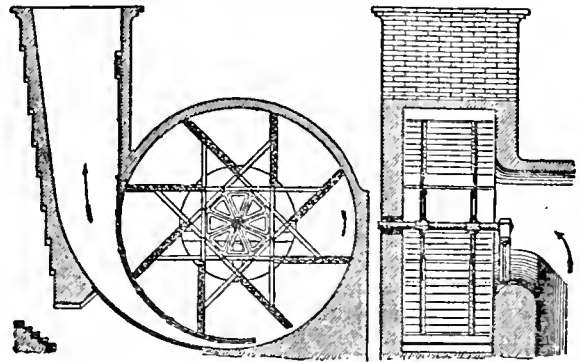
FIG. 12.—Guibal Fan.
