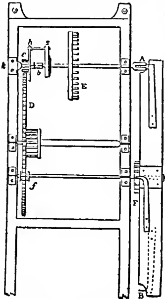
FIG. 16.—Spring Remontoire.
