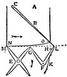
FIG. 13.—Free Escapement.
