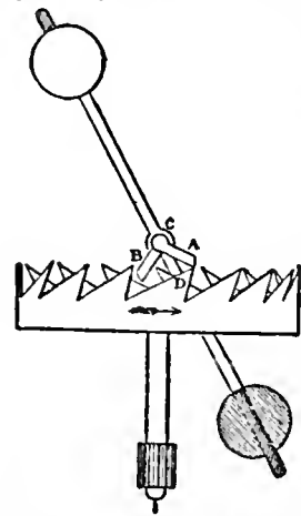
FIG. 1.—Verge Escapement.
