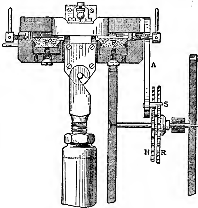
FIG. 11.—Riefler's Escapement.
