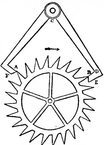
FIG. 9.—Dead Escapement.
