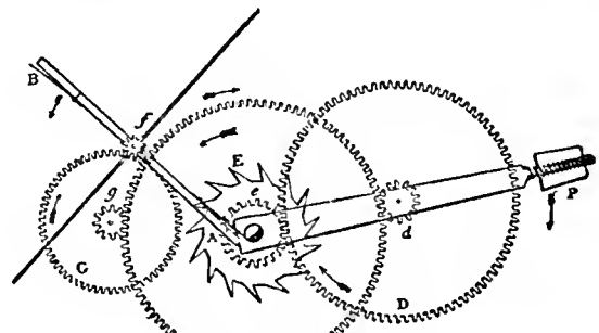
FIG. 15.—Gravity Train Remontoire.
