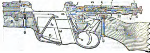
FIG. 13.—Mannlicher, 1895.
