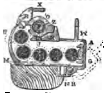
FIG. 17.—Krag-Jørgensen.
