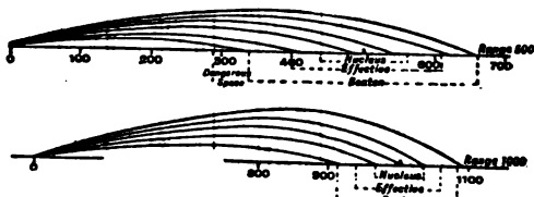
FIG. 19.—Beaten Zone.
