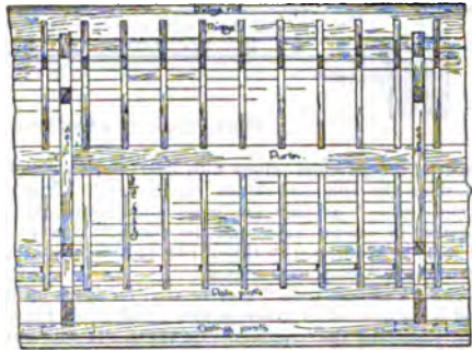
Sectional elevation on AA.
