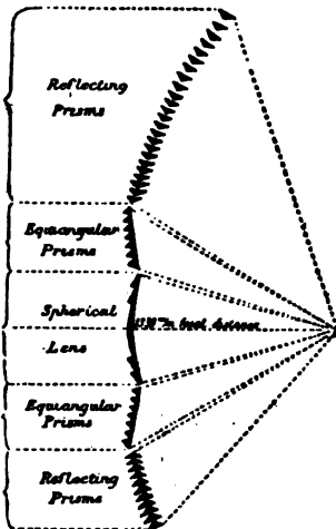
FIG. 40.—Sule Skerry Apparatus.
