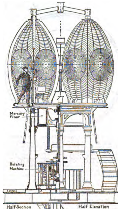
FIG. 43.—Ile Verge Apparatus.
