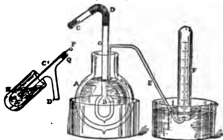
FIG. 13.—Calorimetric Apparatus.
