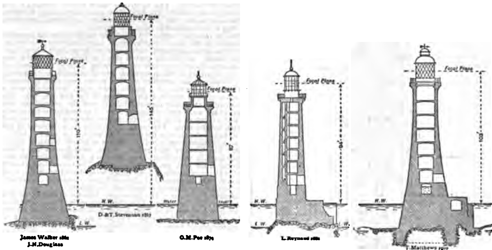
FIG. 14.— Wolf Rock.
