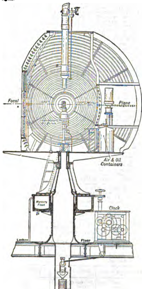
FIG. 42.—Cape Naturaliste Apparatus.
