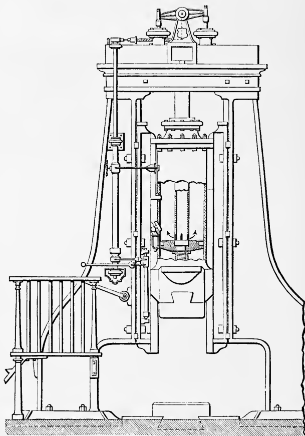
FIG. 45.—Condie's Hammer.
