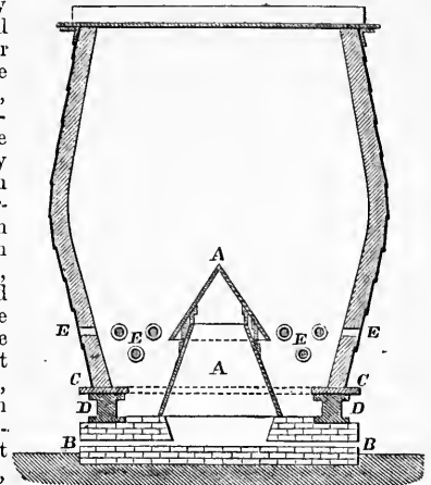
FIG. 1.—Gjers's Kiln.
