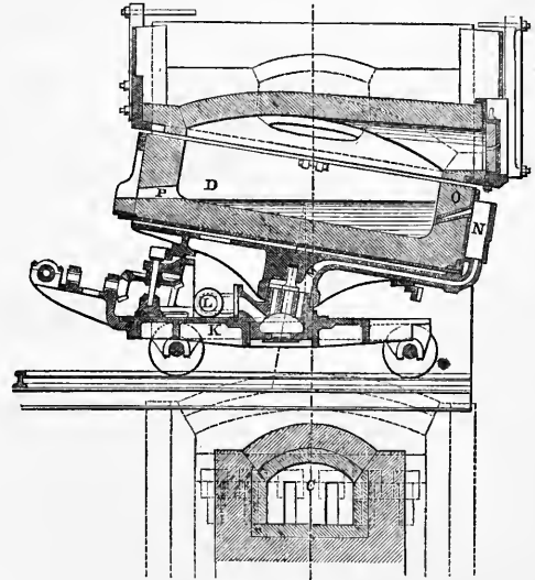
Fig. 63. —Ponsard Forno-Convertisseur—Transverse section.
