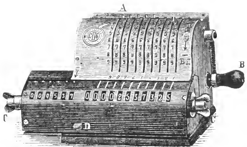
Арифмометръ В. Т. Фернера ОДНЕРЪ
