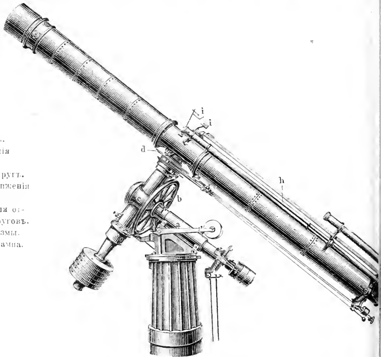
Фиг. 2. Большой рефракторъ Страсбургской Обсерваторіи. Объективъ Мерца въ Мюнхенѣ, механическая часть бр. Реисольдъ въ Лейпцигѣ. Диаметръ объектива 48,7 сант., фокусное разстояніе 7 метровъ.
