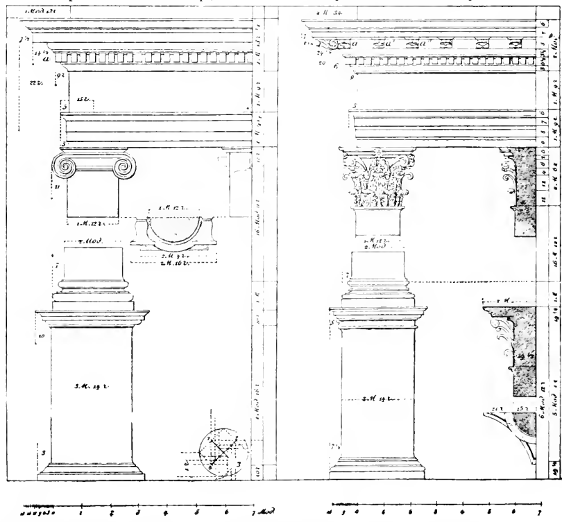
Черт. 14-й. Ионический ордер.
