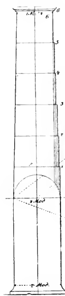
Черт. 10-й Утонение.
