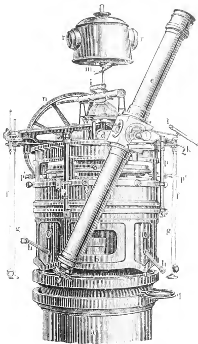
Фиг. 3. Альтазимутъ Страсбургской Обсерватори.
