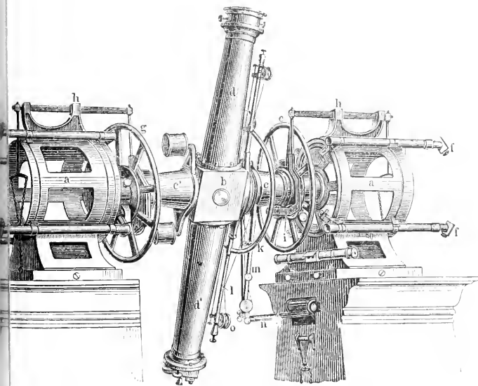
г. Меридіанный кругъ Страсбургской Обсерватори. бр. Ренеольдъ въ Гамбургѣ, объективъ Мерца въ Мюнхенѣ, отверстіе объектива 16,5 сантим., фокусное разстояніе 1,9 метра.
