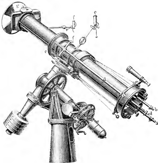
Фиг. 3. Гелиометръ Обсерваторіи въ Нью Гавенѣ (Сѣв. Ам.). Построенъ бр. Реисольдъ въ Гамбургѣ.
