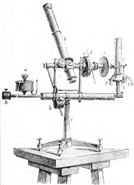
Фотометръ Цельнера (Къ ст. „Астрофотометрія“).
