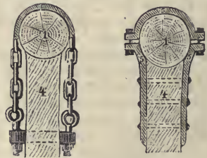
Крѣпленіе Б. съ фортштевнемъ.
