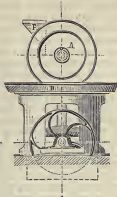
бѣгуны, видъ сбоку.
