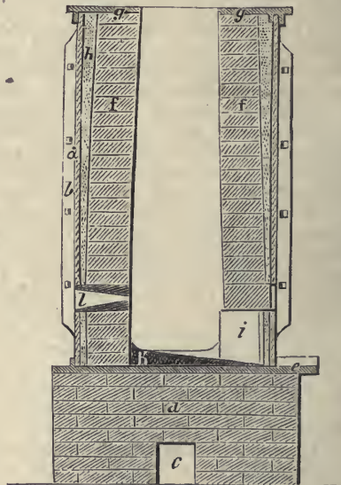
Вагранка, вертикальный разрѣзъ.
