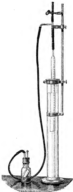
FIG. 41.—Dupré's urea apparatus.
