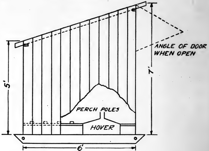
END ELEVATION
