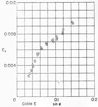
Figure 4e - Cable E, 1/8-inch
