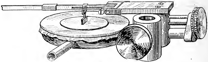
Fig. 13.—Marey tambour.
