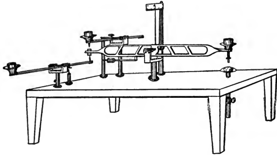
FIG. 29. Zimmermann, 1903, Mk. 280.
