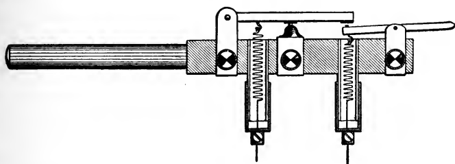
FIG. 49. Ewald's rocking key. See Dumreicher, Zur Messung d. Reactionszeit , 1889, Fig. 5.
