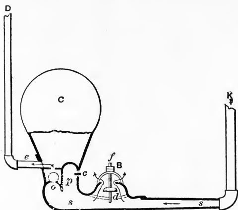
FIG. 159.—HYDRAULIC RAM.
