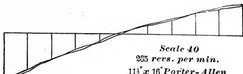
FIG. 293.—INERTIA-DIAGRAM.
