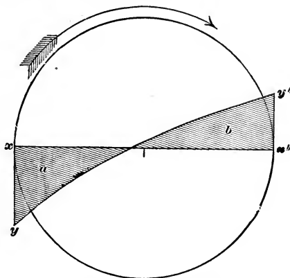
FIG. 296.—INERTIA-DIAGRAM.
