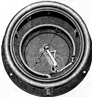
FIG. 171.—BOURDON GAUGE.
