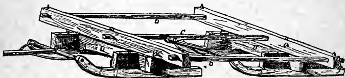
Fig. 44.—MICHIGAN SLED.
