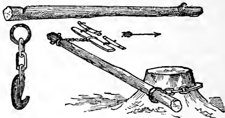
Fig. 176.—A SIMPLE STUMP-PULLER.
