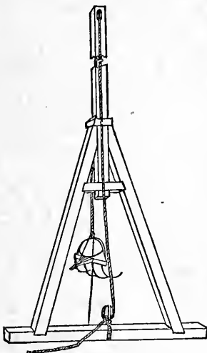
Fig. 153.—HAY DERRICK.
