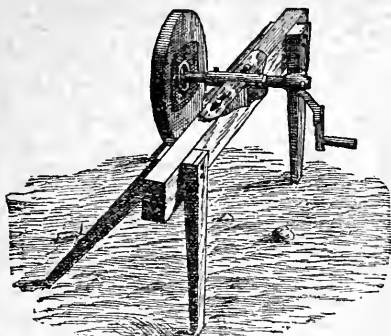
Fig. 71.—GRINDSTONE FRAME.
