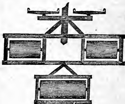
Fig. 47.—A TRIPLE LAND ROLLER.
