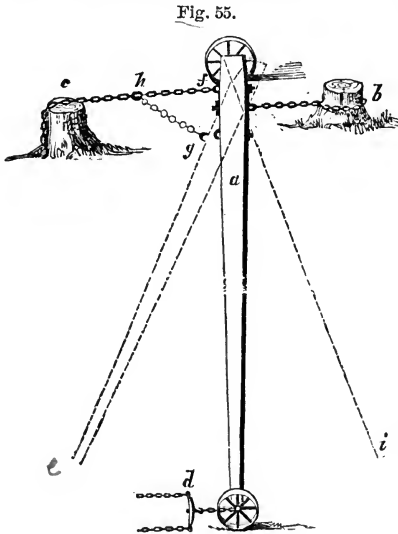
Lever Stump Machine.
