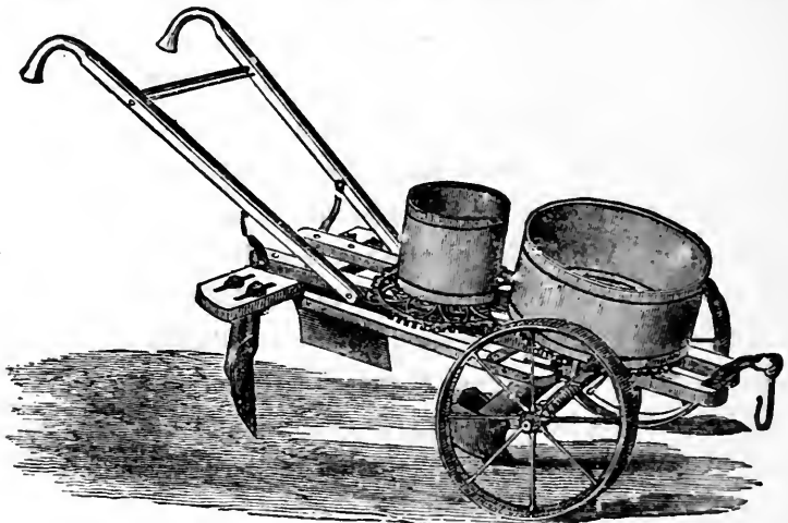
FIG. 33.—TRUE'S POTATO-PLANTER.
