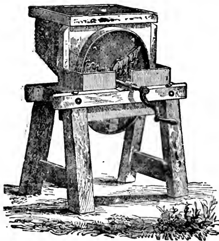
FIG. 77.—ROOT-CUTTER.
