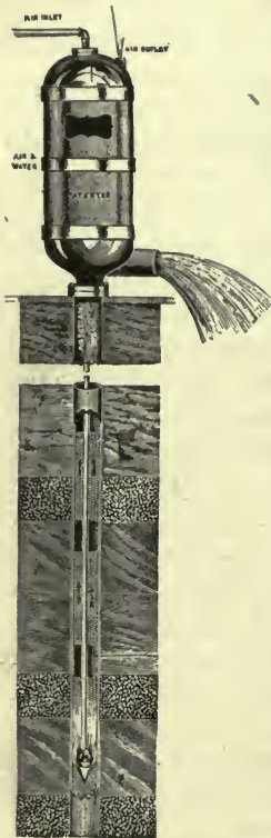
FIG. 90. AIR COMPRESSOR.
